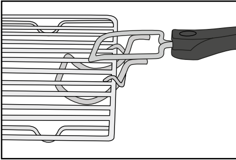
Fig. 1: Aggancio della pinza ⑩ alla griglia ⑧
